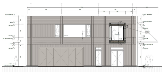
Façade ouest
