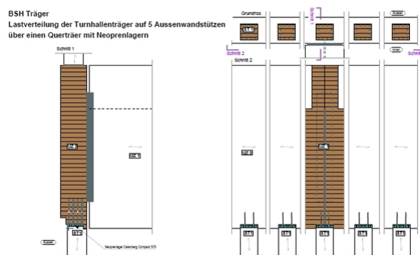
Poutrelles BSH
