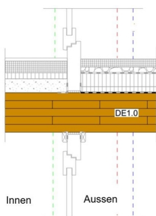
Detail durchlaufende Platte. Bodenaufbau mit 70mm Schüttung, 30mm Trittschalldämmung und 60mm UB
