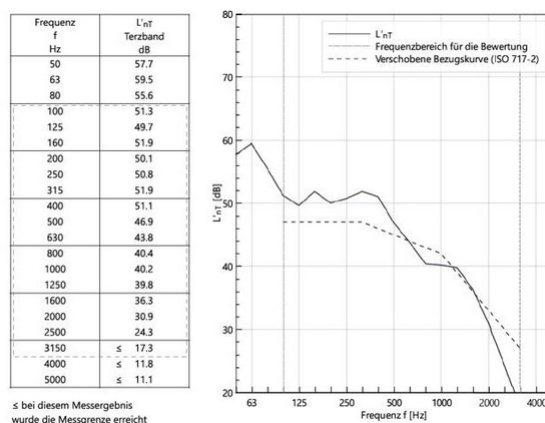
Mit diesem Bodenaufbau wird ein bewerteter Trittschallpegel von L'_{nt}=45\text{dB} nach ISO 717-2 erreicht
