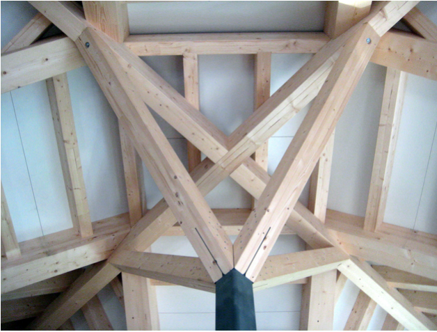
Dachkonstruktion 2
